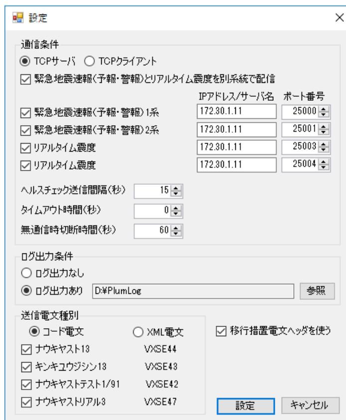
図 2-5: 設定ダイアログ
